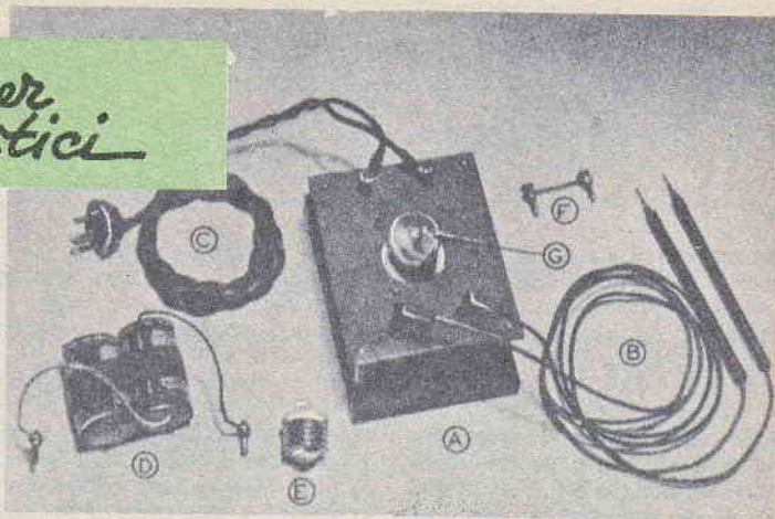
Ecco tutte le parti, basiche ed accessorie dello strumento di prova con le lettere di riferimento
