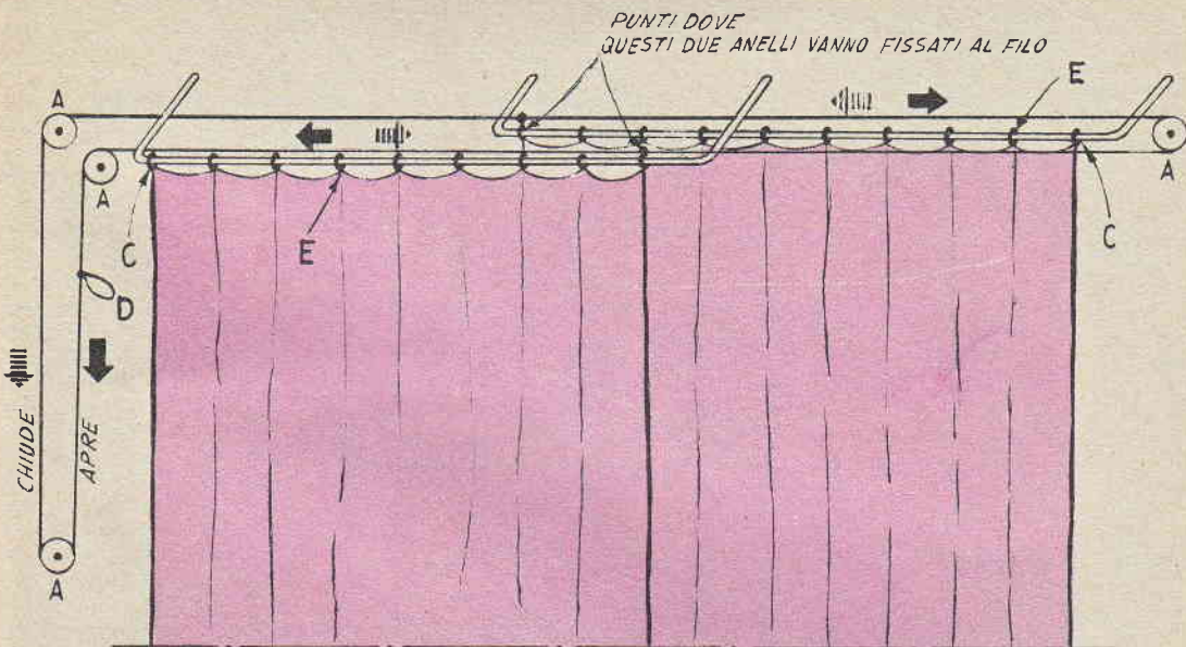
A = PULEGGIE GUIDA FILO ; B = ASTE RICAVATE DA FILO DI METALLO ; C = ANELLI TENUTI FISSI SULLE ASTE ; D = MANIGLIA ANELLO FISSATO AL FILO ; E = ANELLI SCORREVOLI DI OTTONE O FERRO
