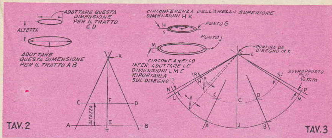
Tavola 2 - Procedimento per la copertura di un paralume tronconico. 1), Tracciare la linea A-B. 2), Tracciare la linea O-Y perpendicolare e centrata rispetto alla prima. 3), Trovare l'altezza e disegnare quindi il segmento C-D. 4), Tracciare poi le diagonali tra A e C e tra B e D, che si incrociano nel punto X. Adottare naturalmente del disegno superiore le dimensioni rilevate dalla struttura metallica del paralume che si intende coprire, seguendo le istruzioni fornite a lato della figura stessa. Tav. 3 - 5), ancorare una puntina da disegno, nel punto X un pezzetto di filo di nylon e poi con centro in X e raggio X-C tracciare la porzione di circonferenza, R-S. 6), sempre con centro in X ma con raggio X-A, tracciare la seconda porzione di circonferenza, ossia la N-P. 7), prolungare verso il basso la linea O-Y, sino a farle incontrare la curva N-P, nel punto che chiameremo J. 8), operare similmente e contrassegnare con la lettera G, il punto di incontro tra la linea perpendicolare centrale e la curva R-S. 9), tracciare le linee X-N ed X-P. 10), tagliare il modello di carta seguendo i punti NRSP, dopo di che si sarà ottenuto il modello in carta avente una precisione più che sufficiente, adatto alle caratteristiche della struttura metallica che si deve coprire.
