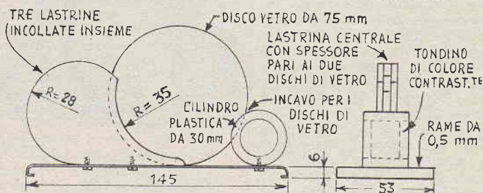
DETTAGLI COSTRUTTIVI PORTAFOTO NELLA SECONDA VERSIONE
