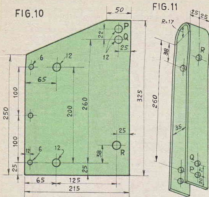
Fig. 10 - Dettagli relativi alla lavorazione delle placche E, in acciaio tenero, Fig. 11 - Dettaglio dell'elemento D, in acciaio tenero
