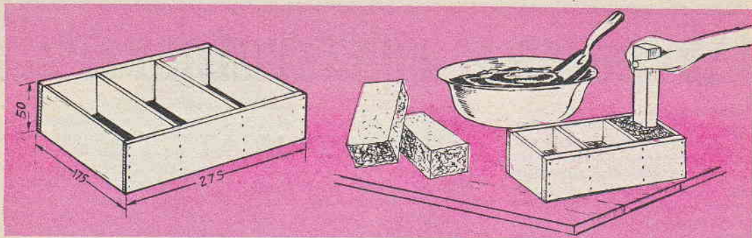
Fig. a Sinistra: Dettagli della forma stampo a tre scompartimenti. Fig. a Destra: Metodo per forzare l'impasto di polvere di carbone nei vari scompartimenti dello stampo e poi estrarre i blocchetti prodotti
