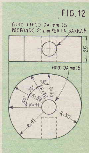
Dettagli per la lavorazione della gamma C, in acciaio tenero
